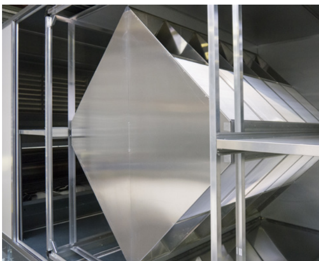
Tegenstroomplatenwisselaar in de unit (tijdens opbouw).
