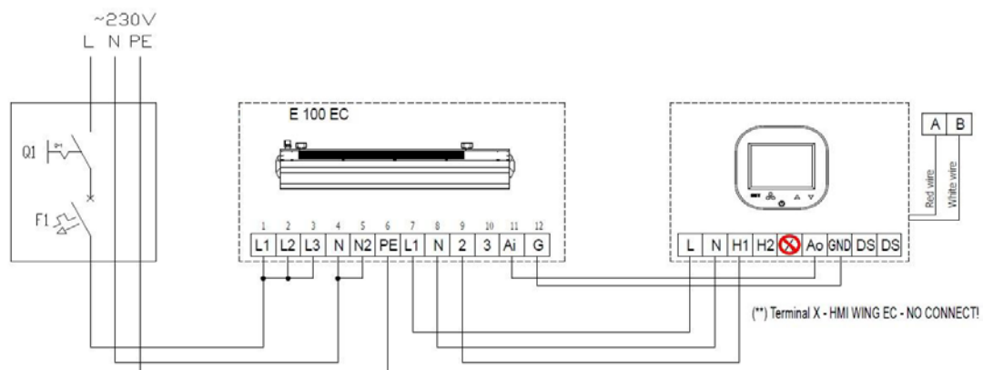
Figuur 3 - EASYAIR E100 aansluiting
