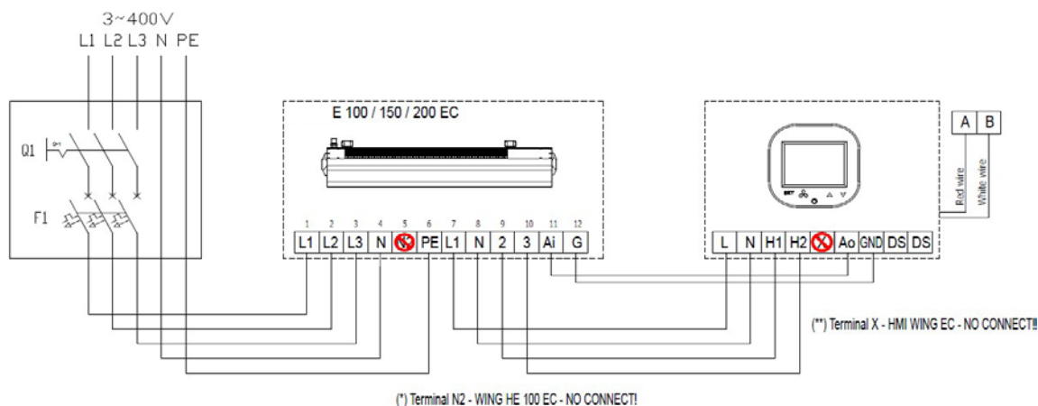
Rys. 1 - Połączenia EASYAIR E100/150/200
