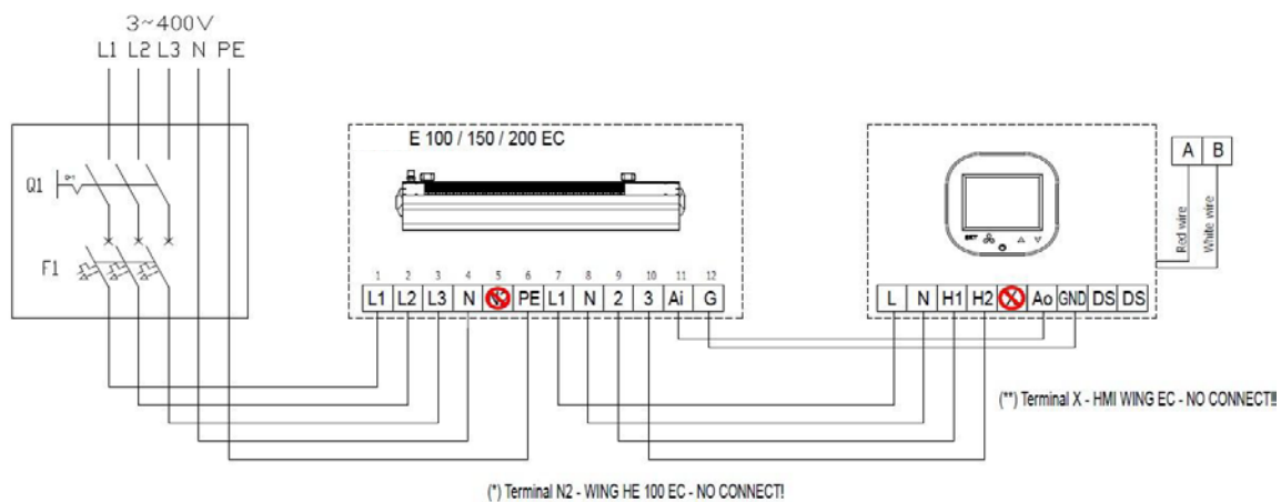
Figuur 2 - EASYAIR E100/150/200 aansluiting
