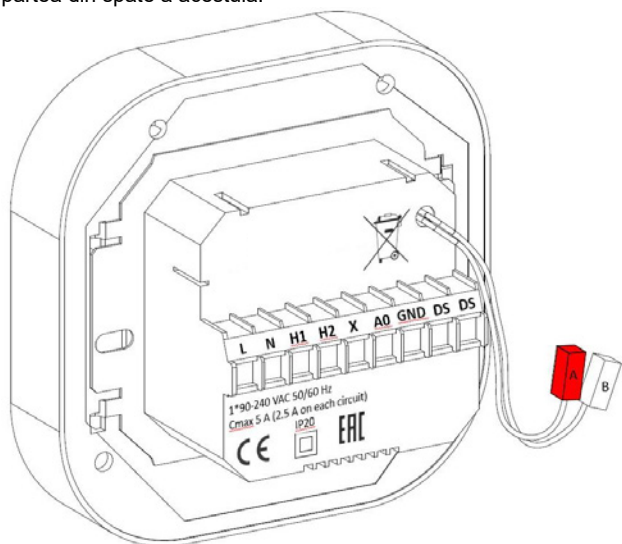
Figura 1 Panoul de conexiuni ale HMI-EC și blocurile terminale
