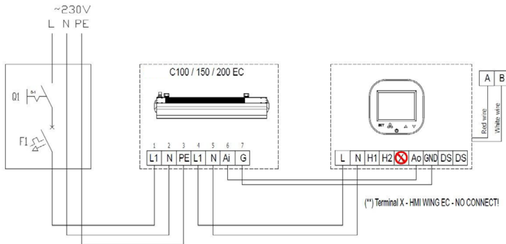
Abbildung 5 - EASYAIR C100/150/200 Anschluss
