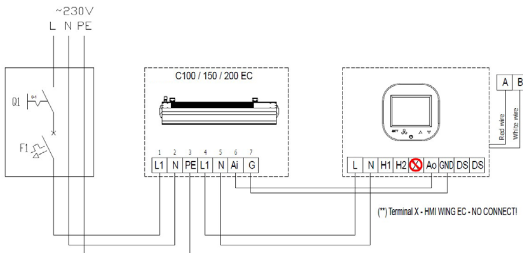
Rys. 5 - EASYAIR C100/150/200
