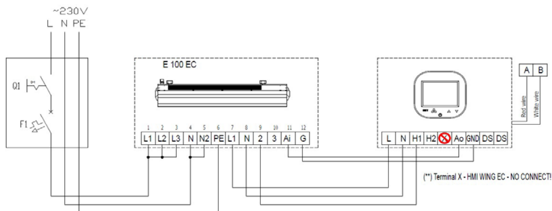
Rys. 2 - Połączenia EASYAIR E100
