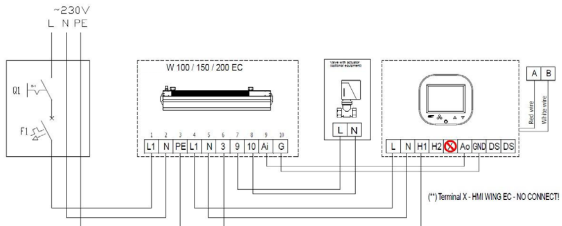
Abbildung 1 - EASYAIR W100/150/200 Anschluss
