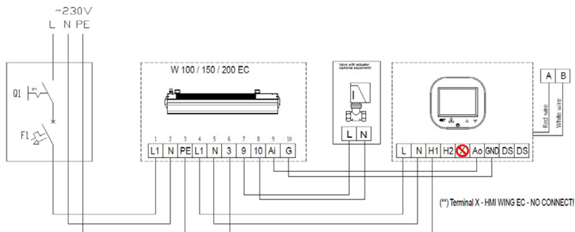
Rys. 2 - Połączenia EASYAIR W100/150/200
