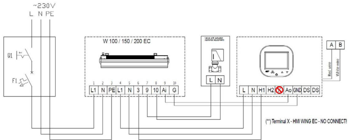
Figuur 1 - EASYAIR W100/150/200 aansluiting
