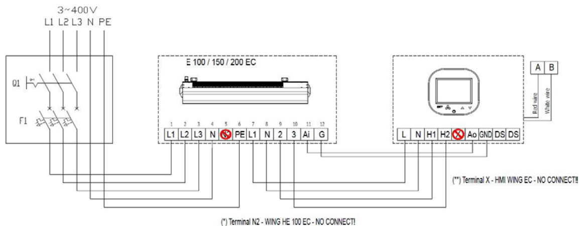
Abbildung 2 - EASYAIR E100/150/200 Anschluss
