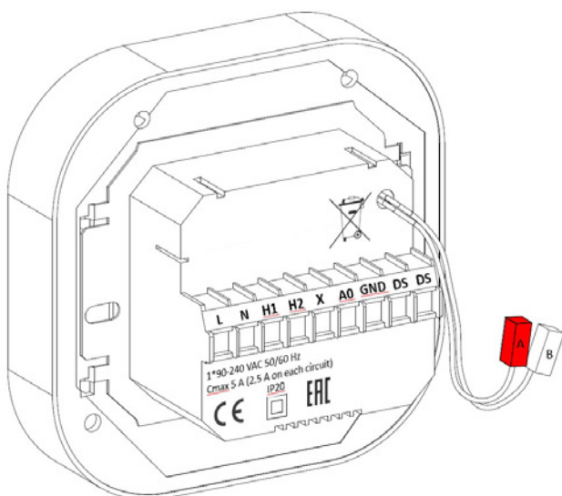
Rys. 1 Panel tylny i zaciski sterownika HMI-EC Funkcja każdego z zacisków wymienionych poniżej:
