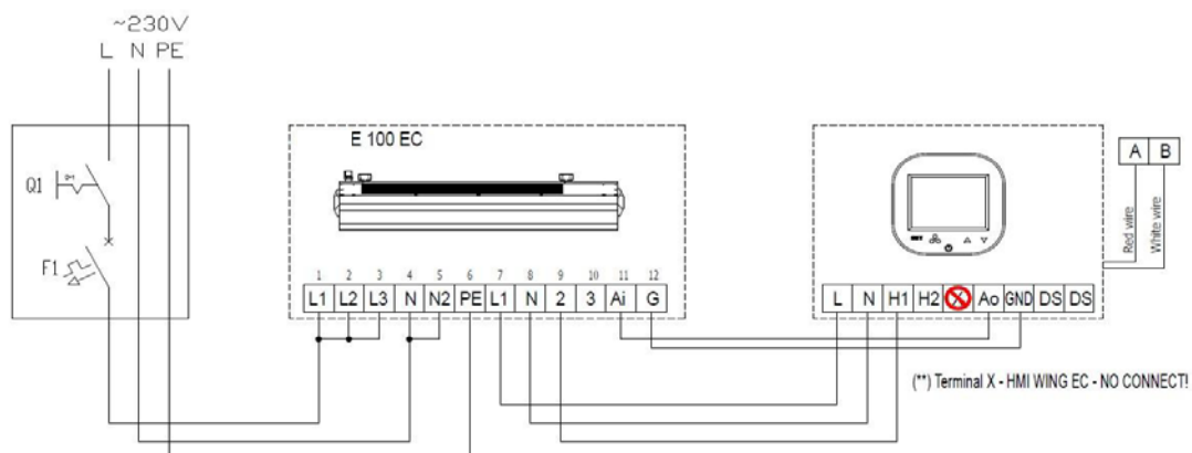
Abbildung 3 - EASYAIR E100 Anschluss.
